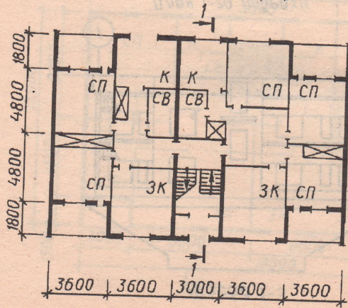
План 1-го поверху
